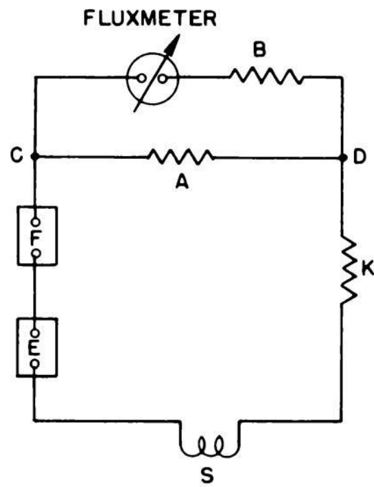
Fig. 2.7—Fluxmeter circuit.
