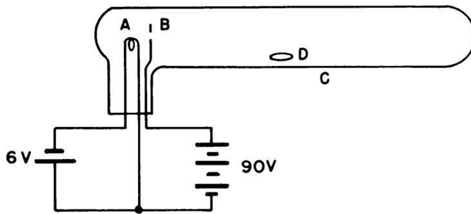
Fig. 2.48—Mercury-arc tube.
